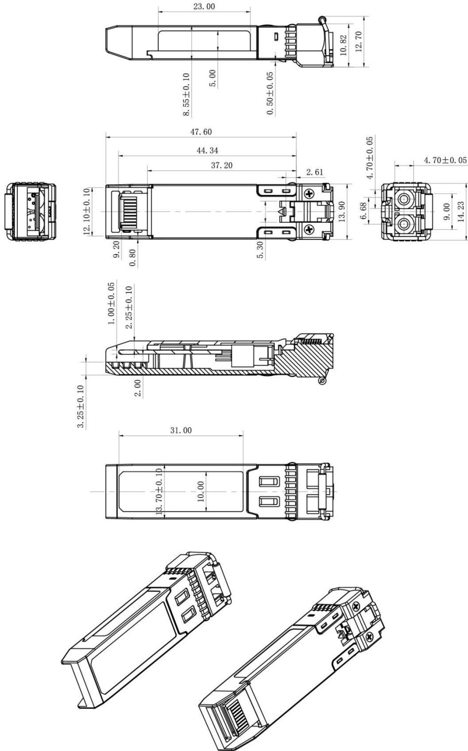
GSFP-SX-D
